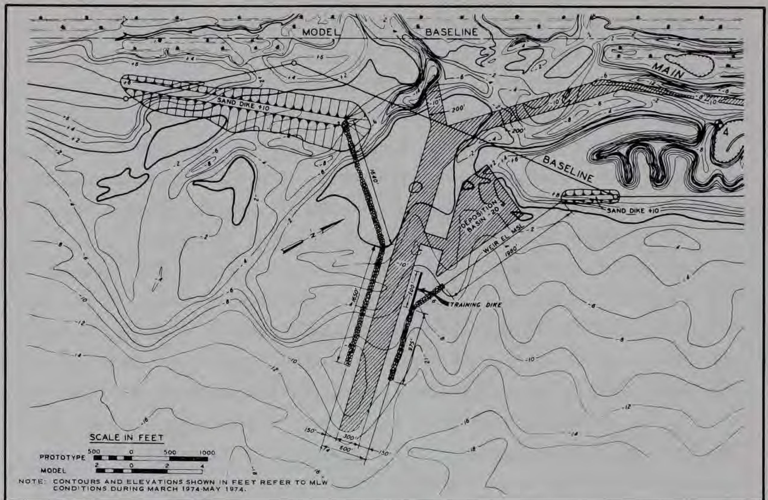
Figure 28. Plan 1E
