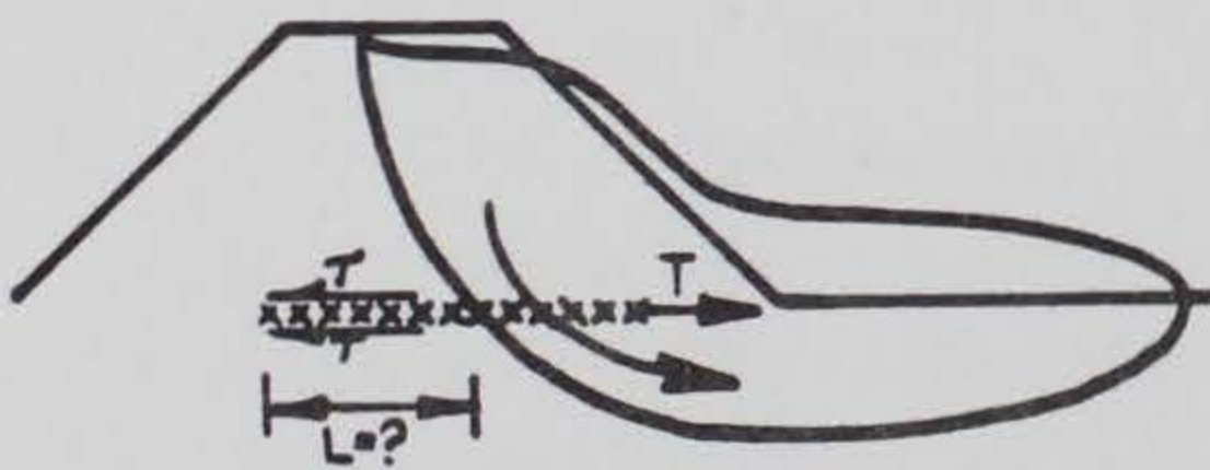
(d) PULLOUT OR ANCHORAGE
